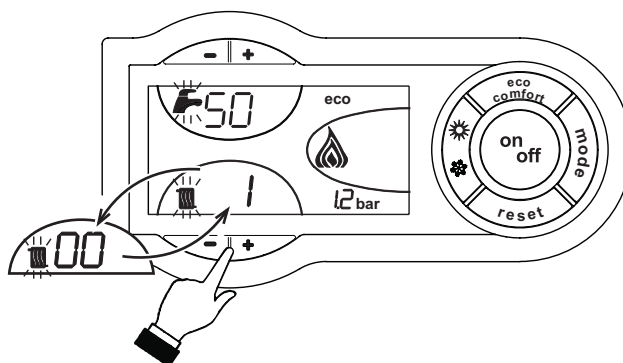
ábra 20 - TEST üzemmód (fűtési teljesítmény = 100%)
