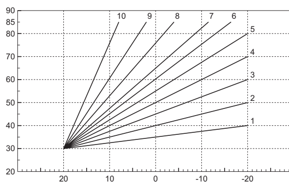
рис. 14 - Компенсационные характеристики
