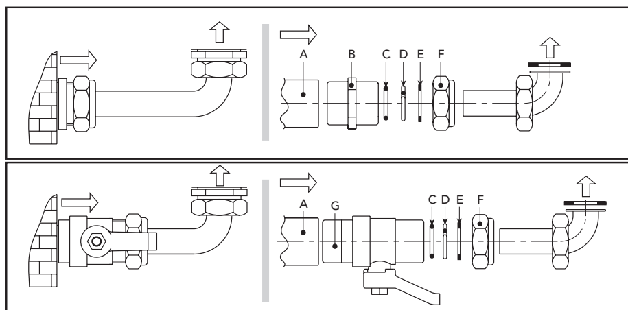
мал. 18 - Комплект з'єднань
