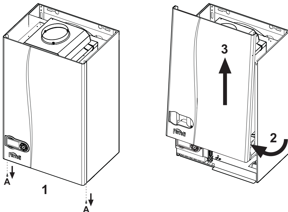
wygląd 22 - Otwieranie płaszcza
