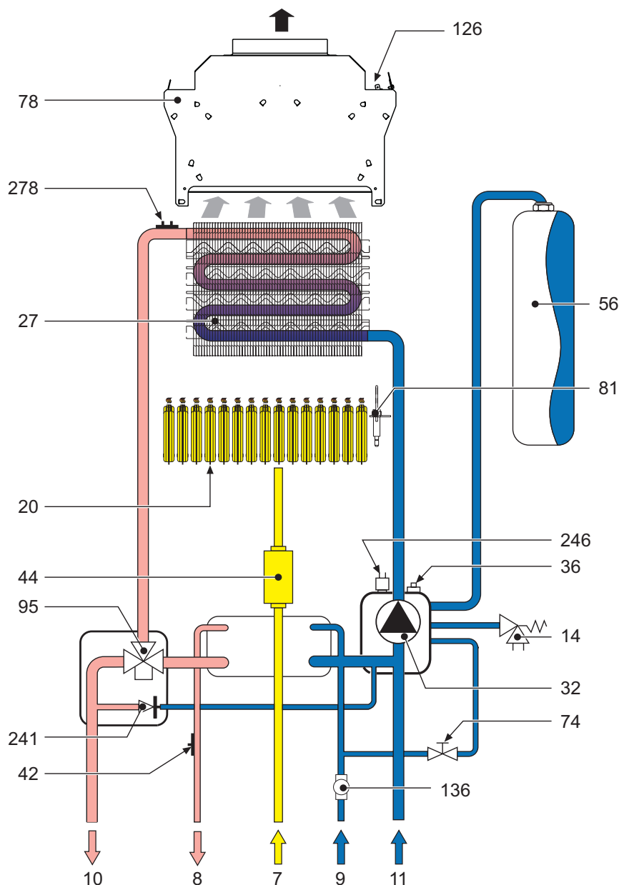
wygląd 25 - Obwód hydrauliczny
