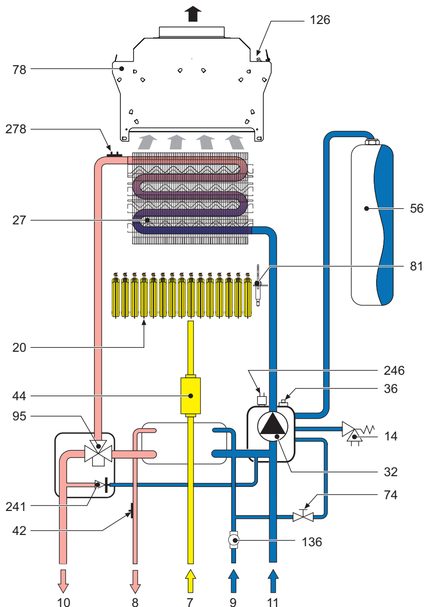
мал. 25 - Гідравлічний контур
