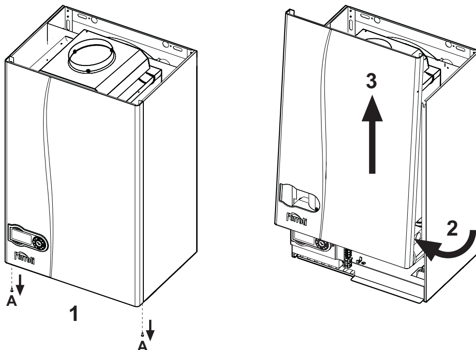
мал. 22 - Зняття кожуха
