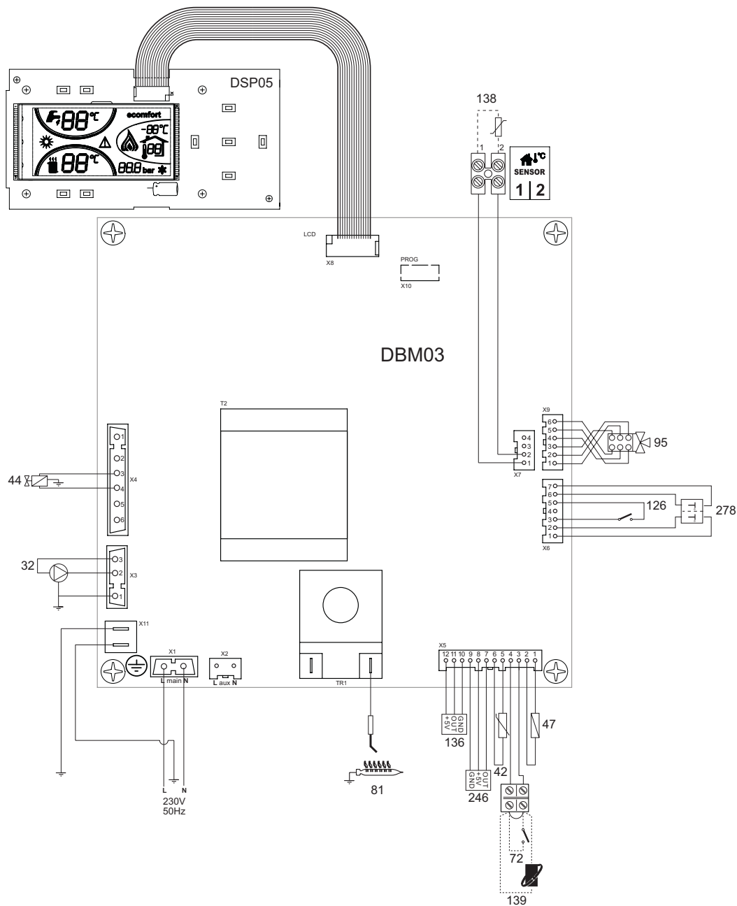
рис. 26 - Электрическая схема
