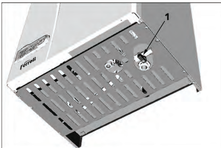
obr. 17 - Plnicí kohout
