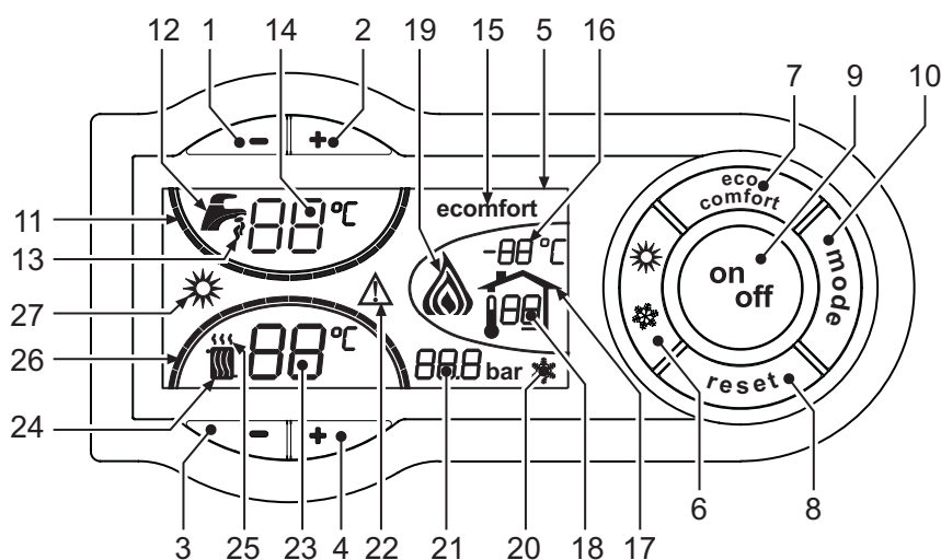
ábra 1 - Vezérlő panel
