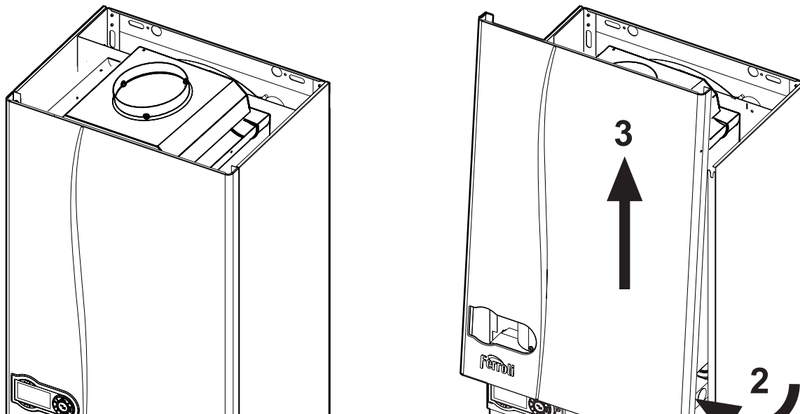
ábra 22 - A köpeny nyitása
