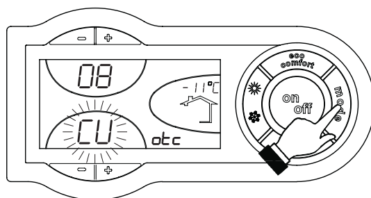
рис. 12 - Компенсационная характеристика
