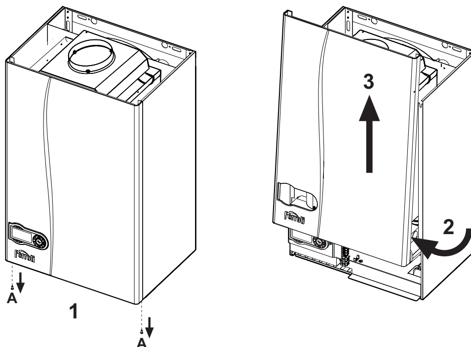
obr. 22 - Otevření pláště
