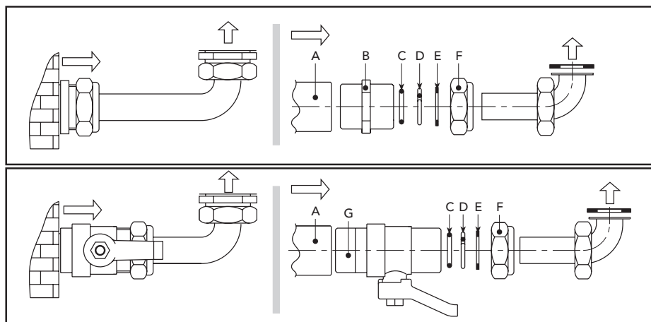
ábra 18 - Csatlakozó készlet
