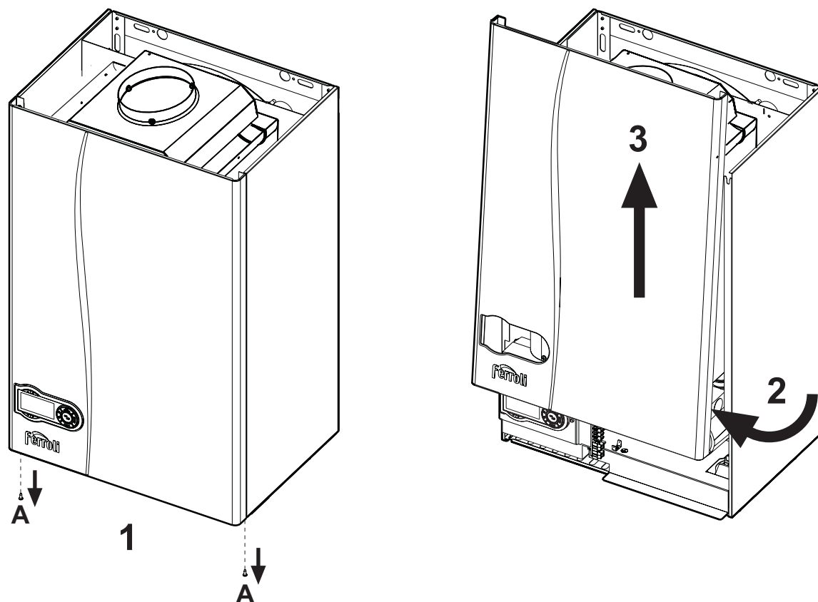
obr. 22 - Otvorenie plášťa
