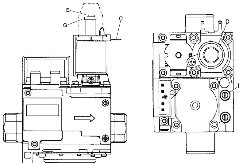
ábra 21 - Gázszelep
