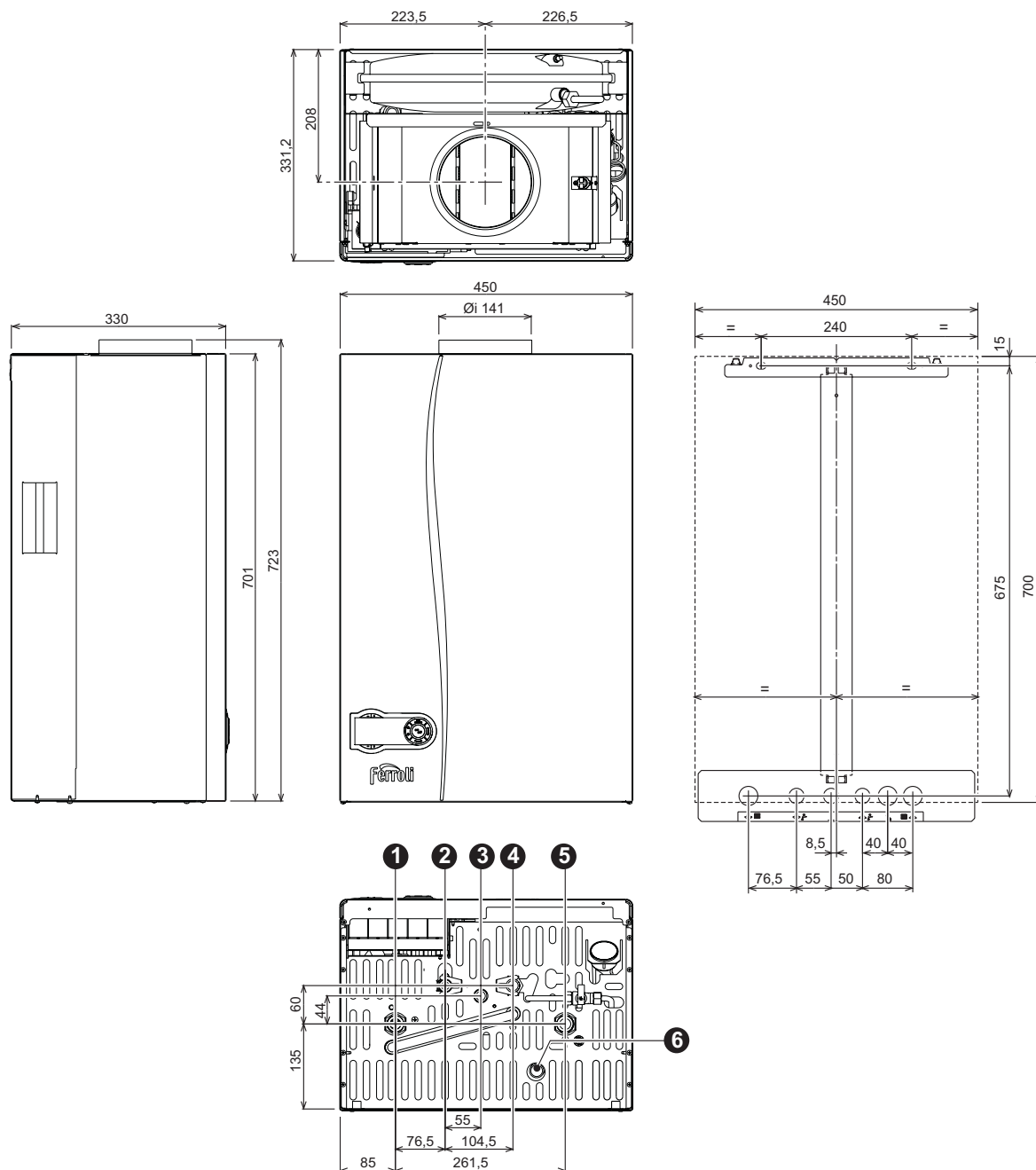
wygląd 23 - Wymiary i złącza
