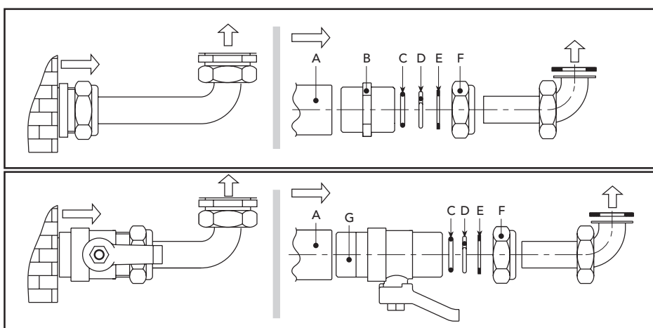
obr. 18 - Souprava k připojení
